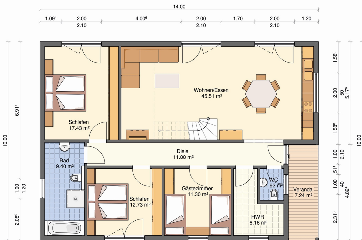
GRUNDRISS Wohnfläche EG=116,94 m 2
