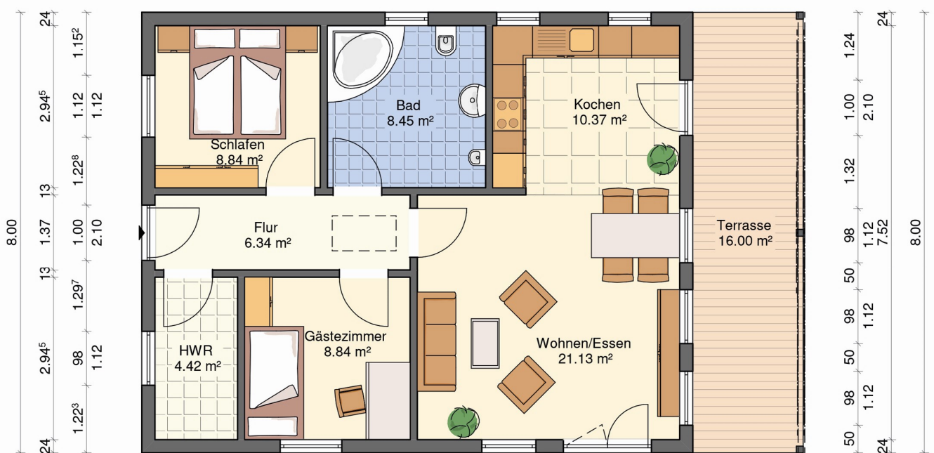
GRUNDRISS Wohnfläche EG= 76,38 m 2
