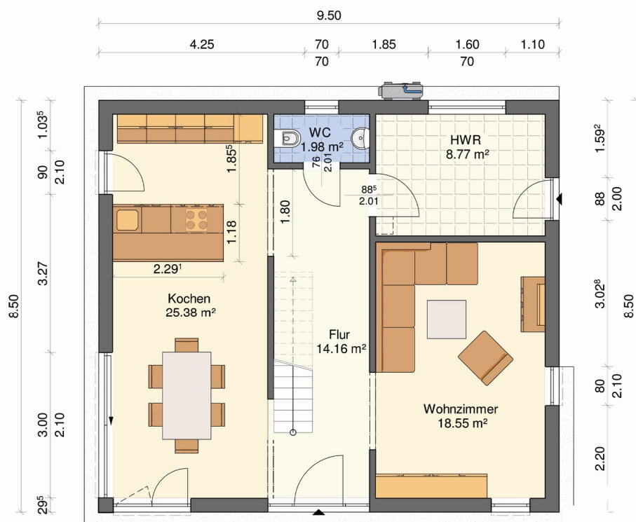
GRUNDRISS Wohnfläche EG= 65,67 m 2
