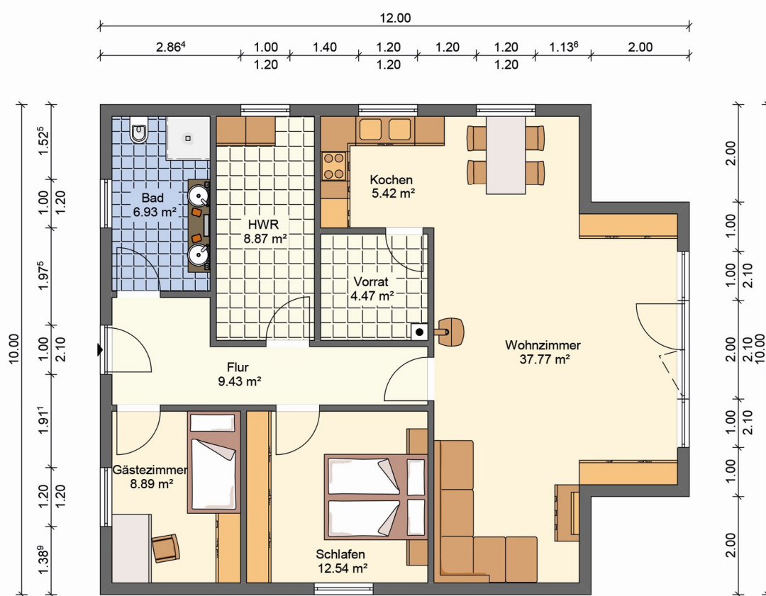
GRUNDRISS Wohnfläche EG= 97,23 m²
