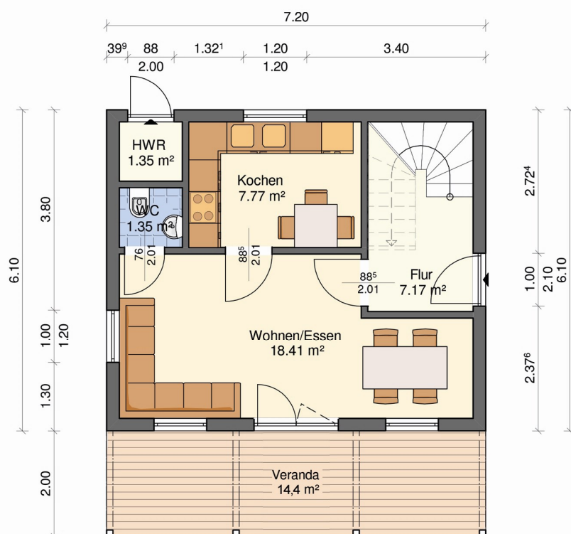
GRUNDRISS Wohnfläche EG= 39,63 m²
