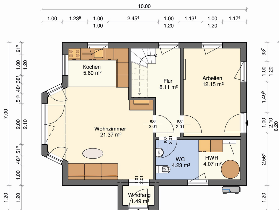
GRUNDRISS Wohnfläche EG= 54,80 m²
