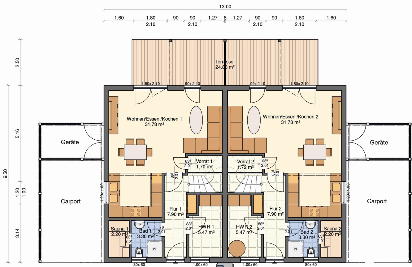
GRUNDRISS Wohnfläche EG= 52,82 m 2 /Wohneinheit
