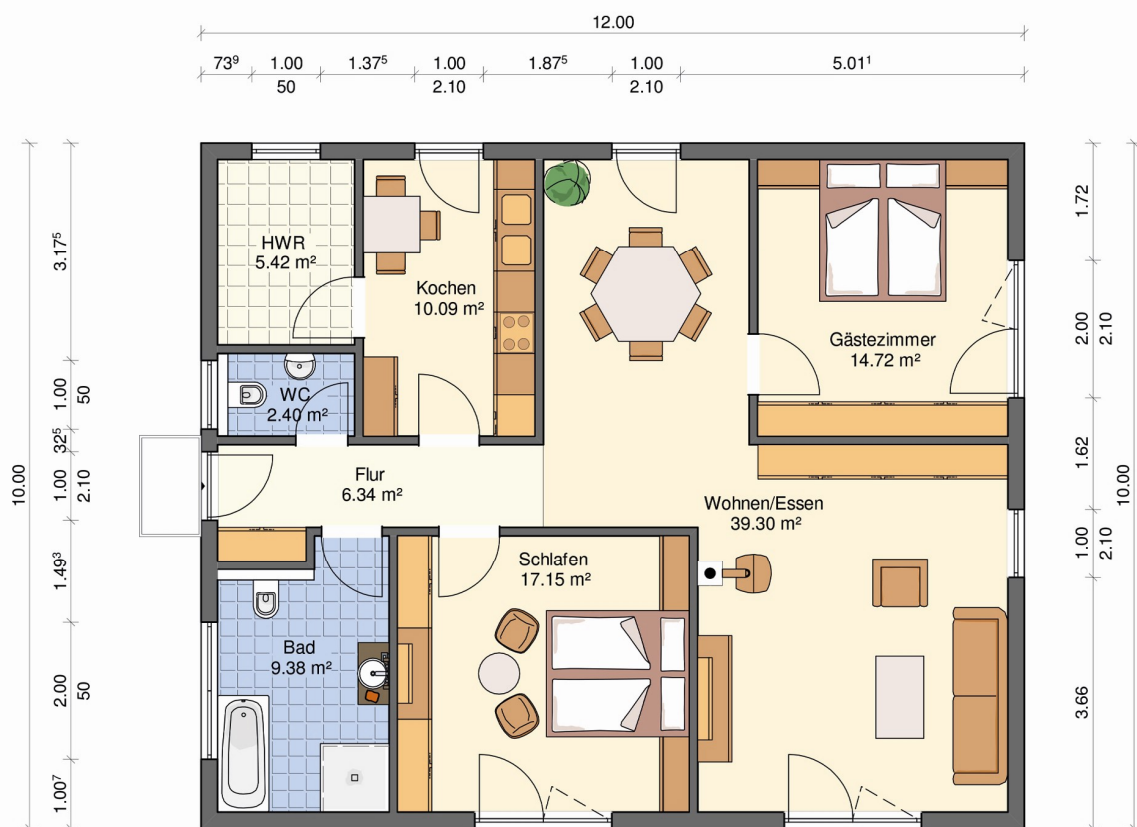
GRUNDRISS Wohnfläche EG=104,8 m 2
