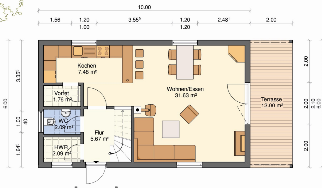
GRUNDRISS Wohnfläche EG=54,55 m²
