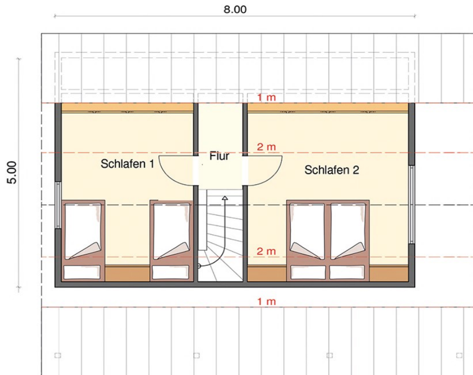
OBERGESCHOSS
