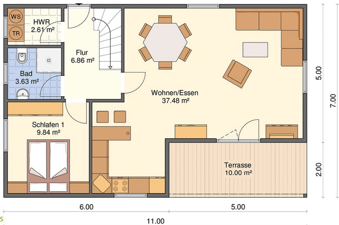
ERDGESCHOSS
