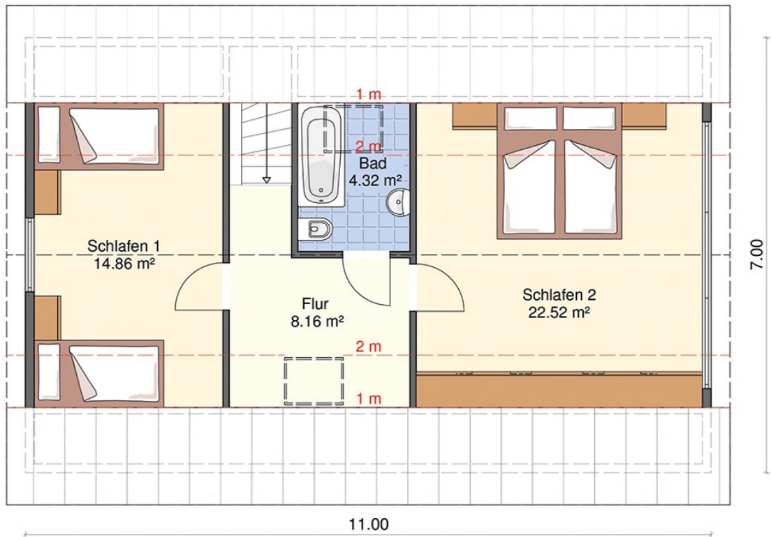
OBERGESCHOSS
