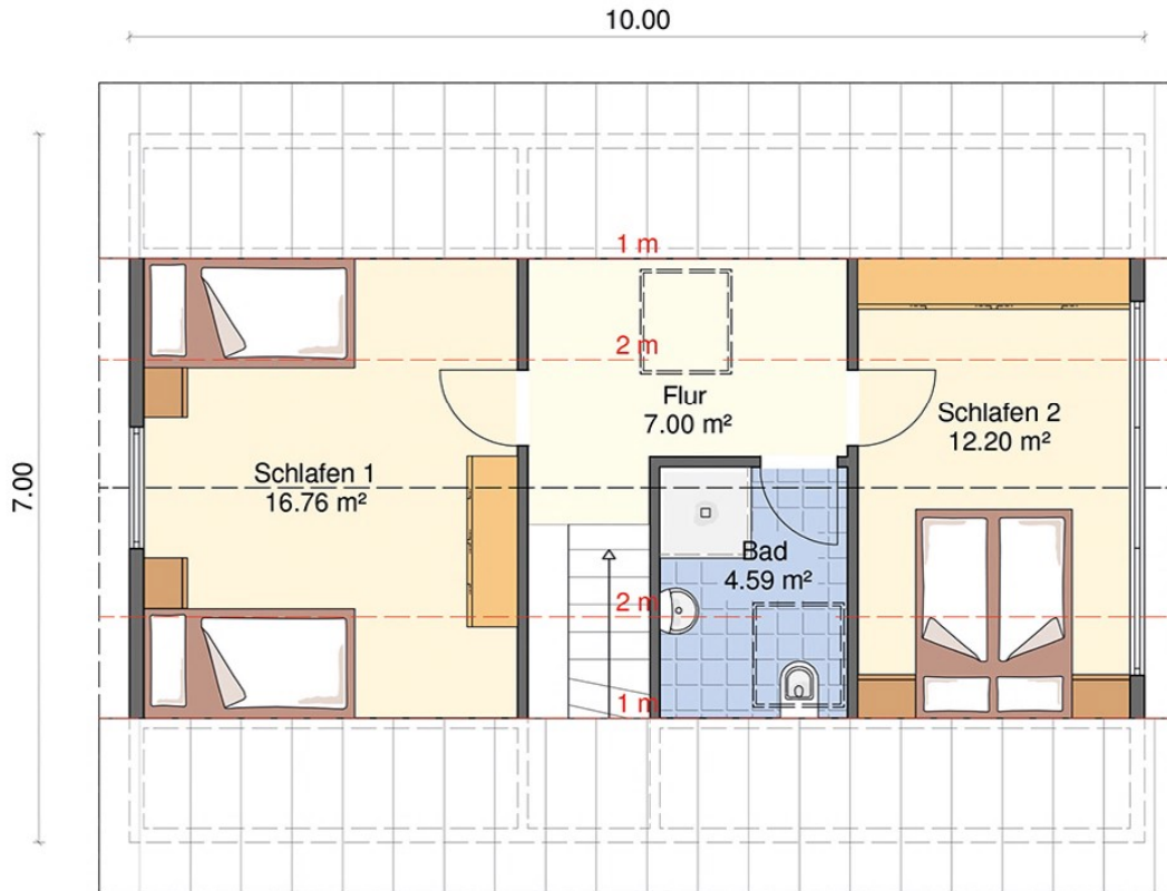
OBERGESCHOSS
