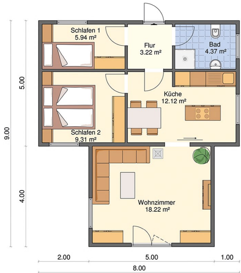
Ausführung eingeschossig als Holzrahmenbau
