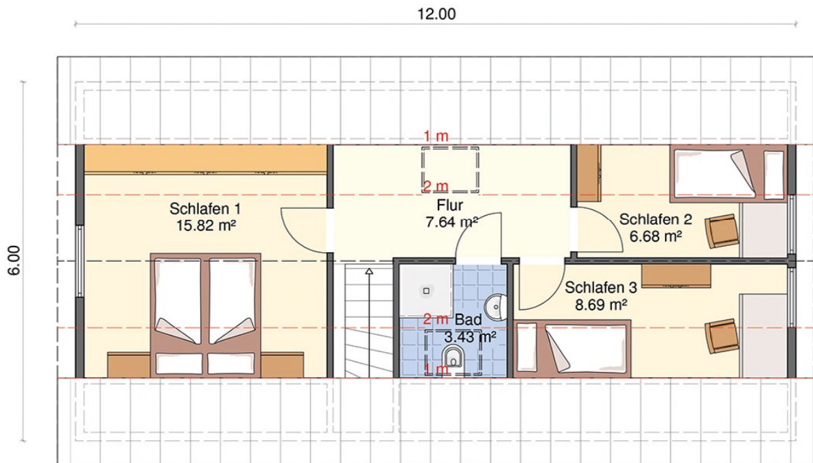
OBERGESCHOSS
