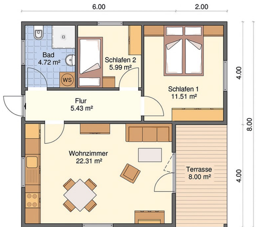
Ausführung eingeschossig als Holzrahmenbau
