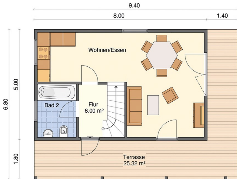
ERDGESCHOSS
