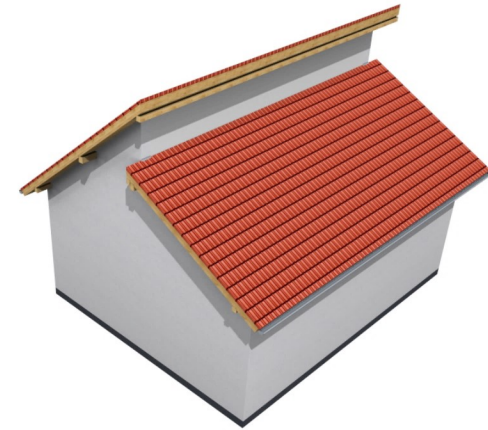
Versetztes Pulldach
